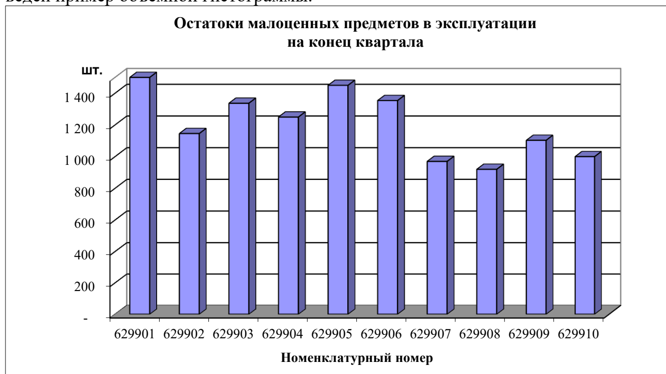
Рис. 1. Гистограмма для анализа остатков малоценных предметов
